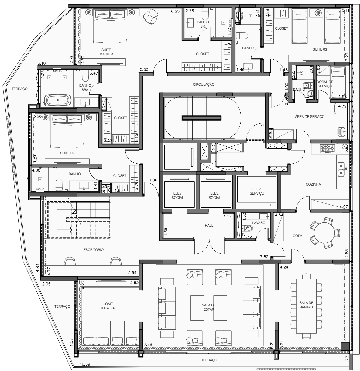
PAVIMENTO INFERIOR
