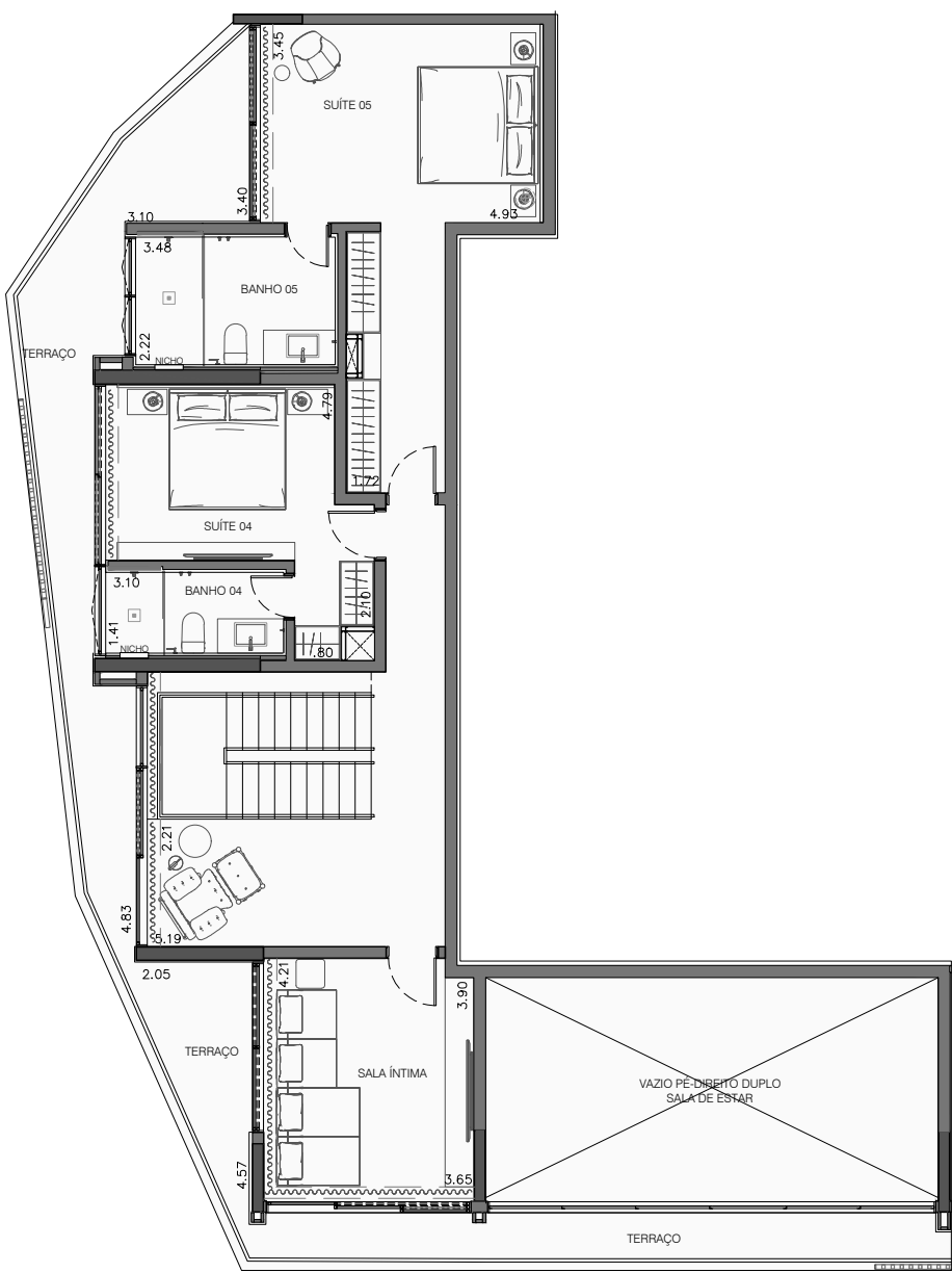
PAVIMENTO SUPERIOR
